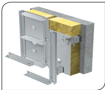
Рис. 19 Общий вид закрепленной панели с внутренней стороны.
