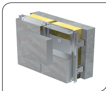
Рис. 20 Общий вид закрепленной панели. Лицевая сторона.
