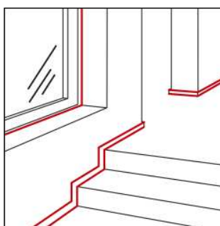
Деформационные швы
