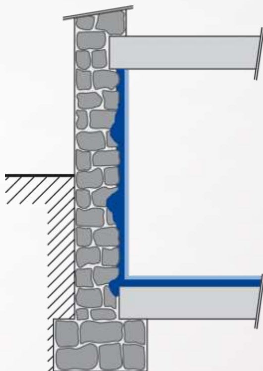
Фундаменты
