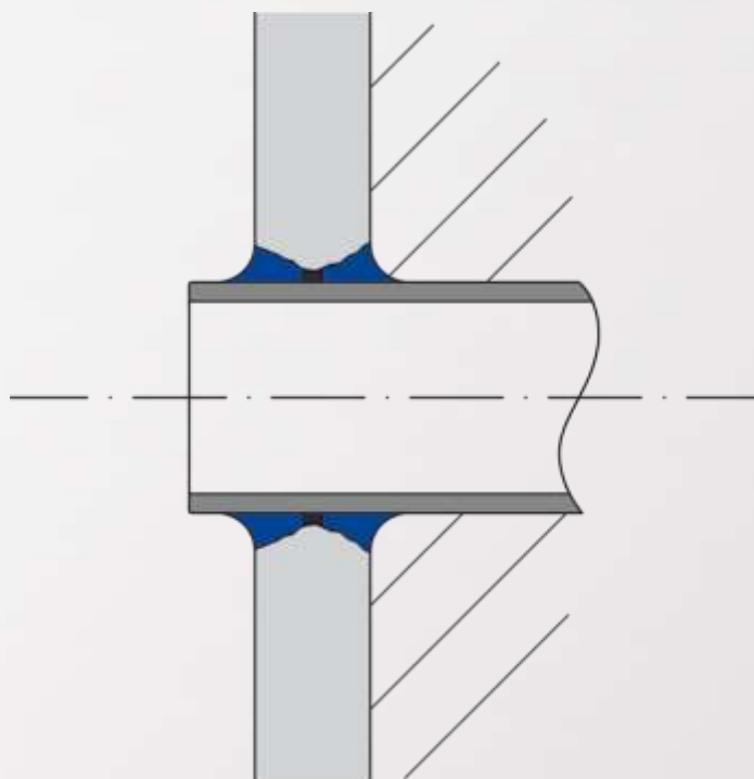
Проходки трубные
